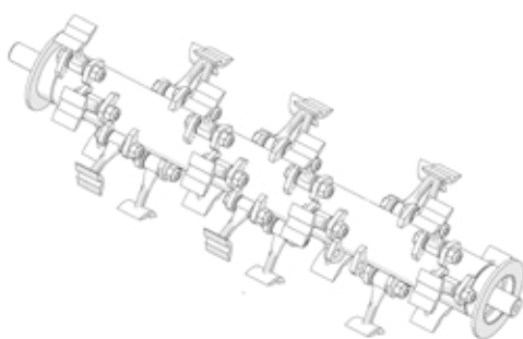
Rotor débroussaillage
